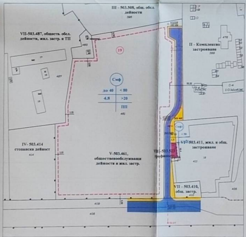
ПЛАН ЗА ЗАСТРОЯВАНЕ М 1:1000
