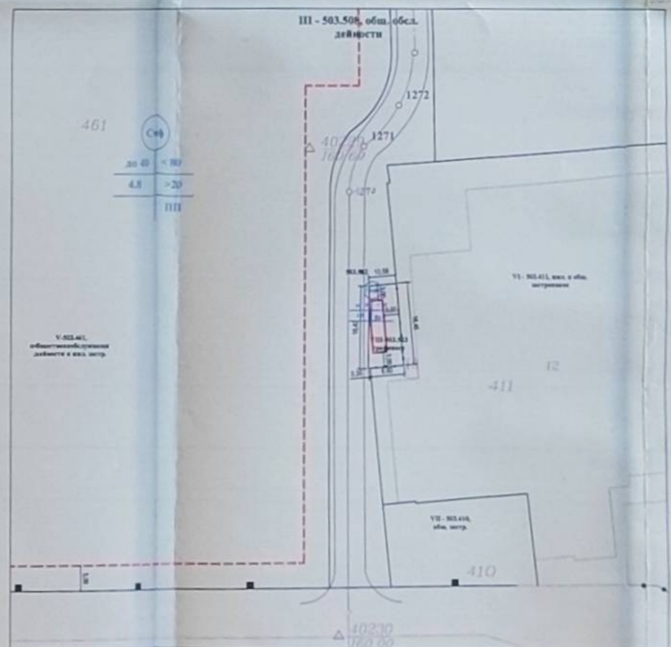
ПЛАН ЗА ЗАСТРОЯВАНЕ М 1:500
