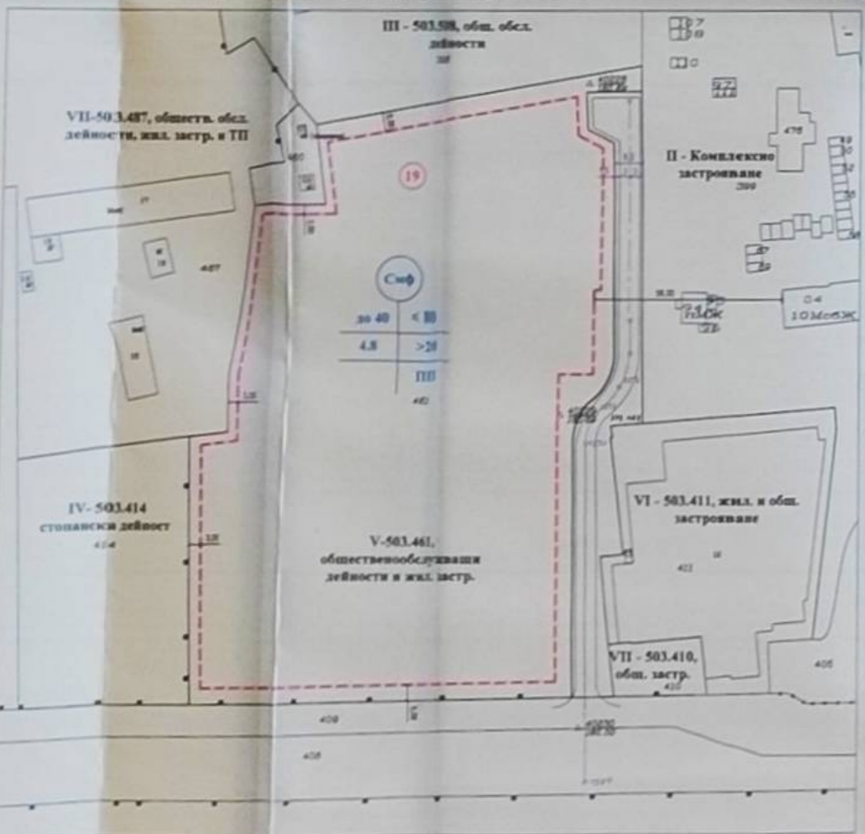
ИЗВАДКА ОТ ПРЗ-ПЛАН ЗА ЗАСТРОЯВАНЕ (Зап. 18 ОА 2670 от 15.11.2018г. Община Пловдив) М 1:1000
