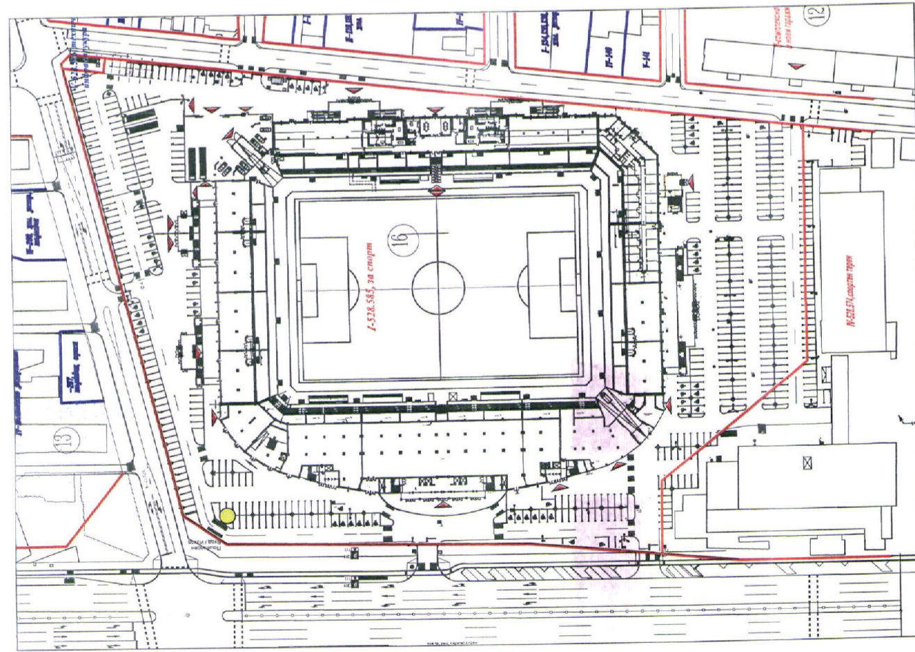
СИТУАЦИЯ М 1:2000
