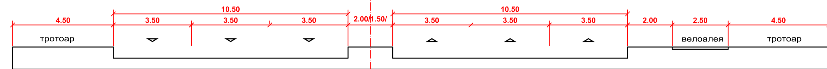
ТИПОВ НАПРЕЧЕН ПРОФИЛ III А КЛАС - 2 x 3
