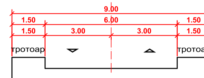
ТИПОВ НАПРЕЧЕН ПРОФИЛ VI Б КЛАС
