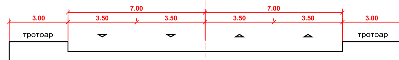
ТИПОВ НАПРЕЧЕН ПРОФИЛ III Б КЛАС - 2 + 2
