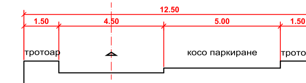
ТИПОВ НАПРЕЧЕН ПРОФИЛ VI Б КЛАС - еднопосочно движение
