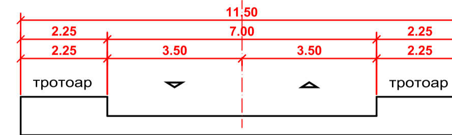
ТИПОВ НАПРЕЧЕН ПРОФИЛ V КЛАС
