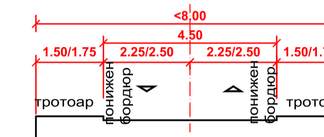
ТИПОВ НАПРЕЧЕН ПРОФИЛ VI Б КЛАС
