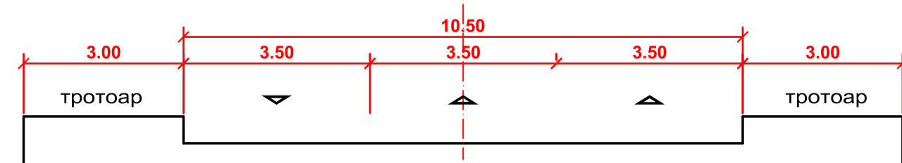
ТИПОВ НАПРЕЧЕН ПРОФИЛ IV КЛАС
