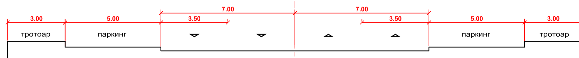
ТИПОВ НАПРЕЧЕН ПРОФИЛ III Б КЛАС - 2 + 2 с паркиране
