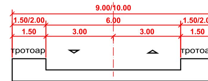
ТИПОВ НАПРЕЧЕН ПРОФИЛ VI А КЛАС
