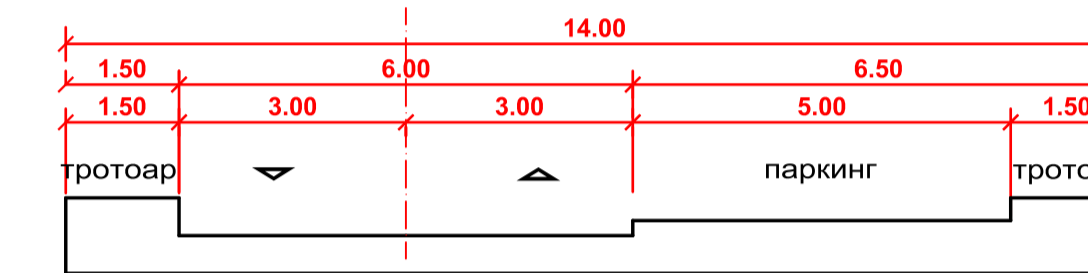
ТИПОВ НАПРЕЧЕН ПРОФИЛ VI А КЛАС
