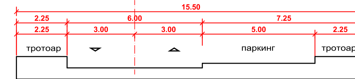
ТИПОВ НАПРЕЧЕН ПРОФИЛ V Б КЛАС - с паркиране
