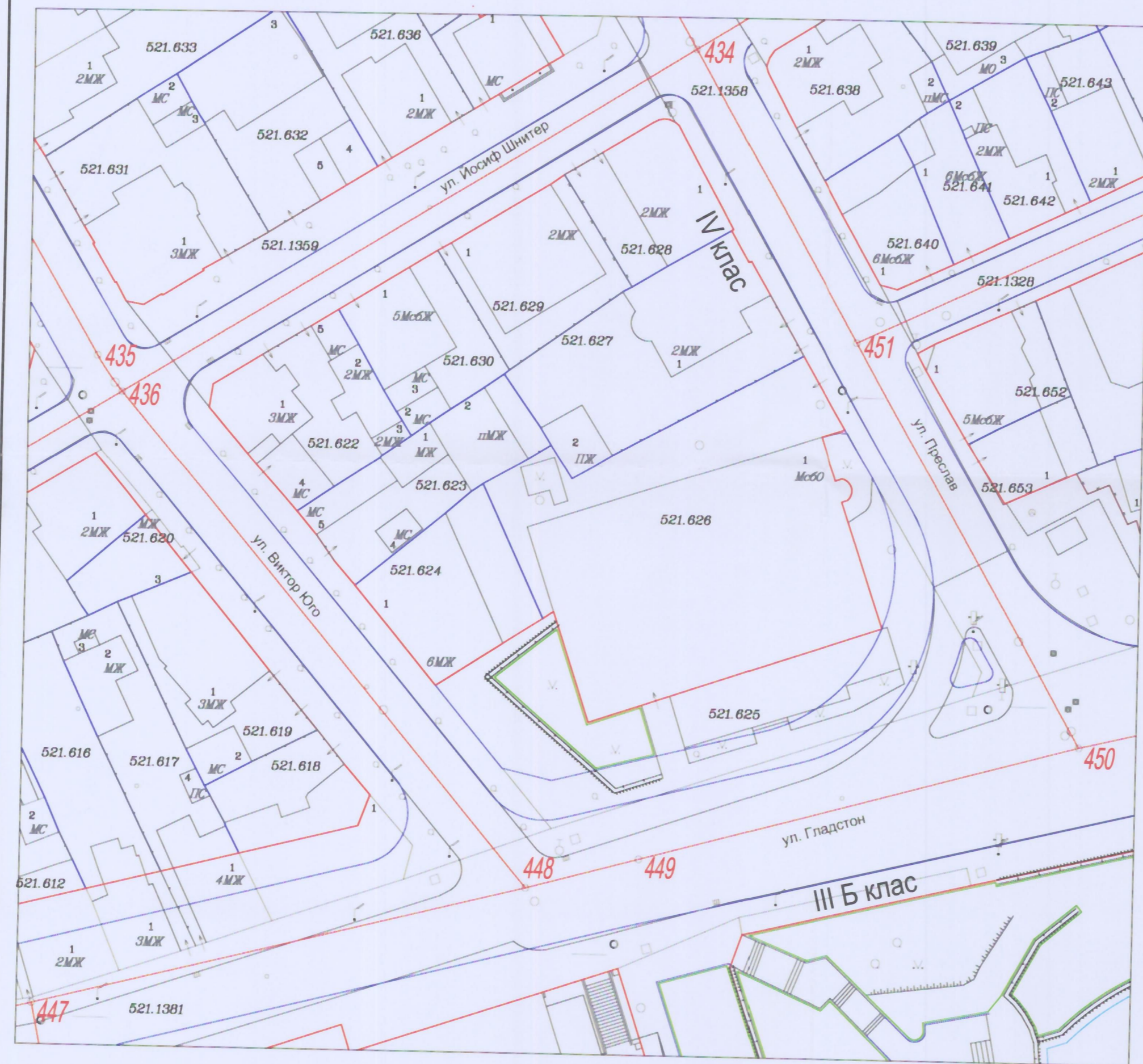
Извадка от предварителен проект ПУП - ПР, Централна градска част, гр. Пловдив, ПП приет с протокол №56, т.1 от 12.120.2014г. на ЕСУТ- Пловдив МАЩАБ 1 : 500
